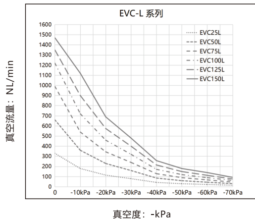
EVC-L 不同真空度 (-kPa)的真空流量(NL/min)
