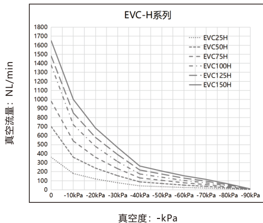
EVC-H 不同真空度 (-kPa)的真空流量(NL/min)
