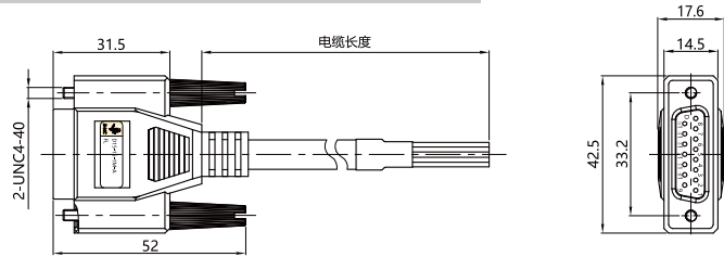
SR系列集成阀组连接器电缆外形图及接线图
