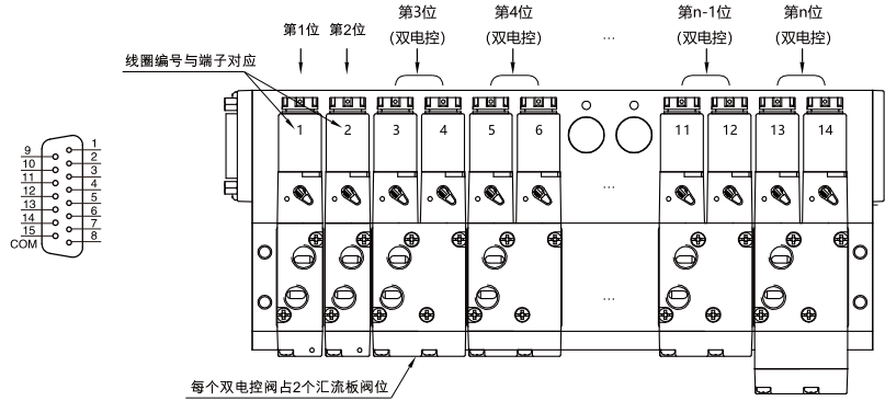
单/双电控混装配线示意图 (双电控最大7位)
