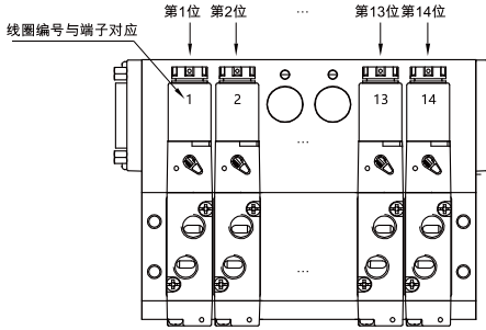
单电控配线示意图 (最大14位)
